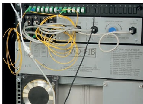
Coupleur optique 4 voies
