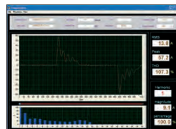
Courant pic - THD - Spectre des harmoniques
