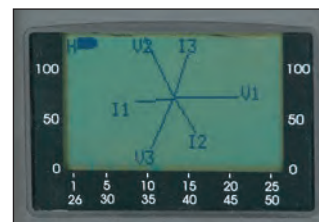
Diagramme des phases en triphasé V1 V2 V3 I1 I2 I3 \varphi
