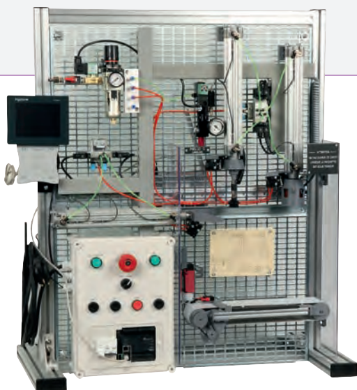
Réf. PNEU23-C
