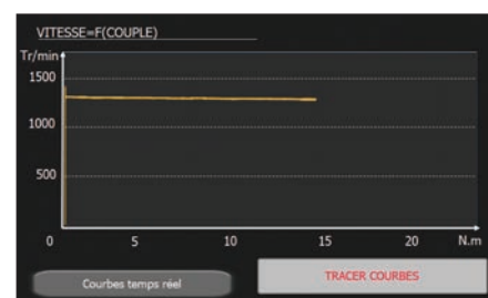
Evolution de la vitesse en fonction du couple
