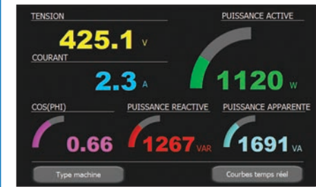
Visualisation pour machine asynchrone mono et tri
