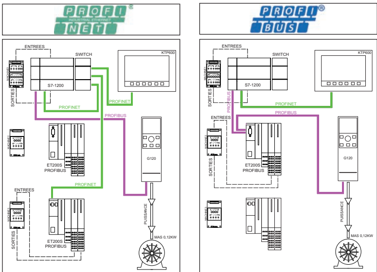
Schémas de câblage et Bus de la version MAQ-NET
