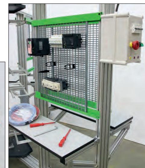
Chaque bras est équipé d'un coffret d'alimentation. Positionné à l'extrémité des bras les plus courts et derrière l'armoire sur le 3ème bras.
