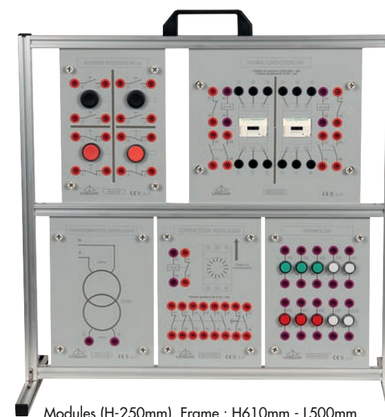
Modules (H-250mm). Frame : H610mm - L500mm.
